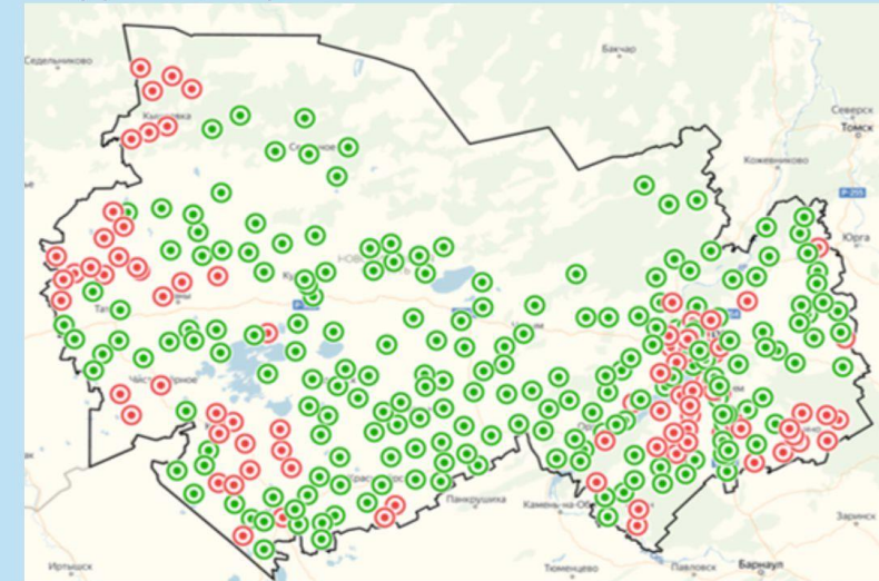
Загрузка центров питания АО «РЭС» на 01.10.2019г.
